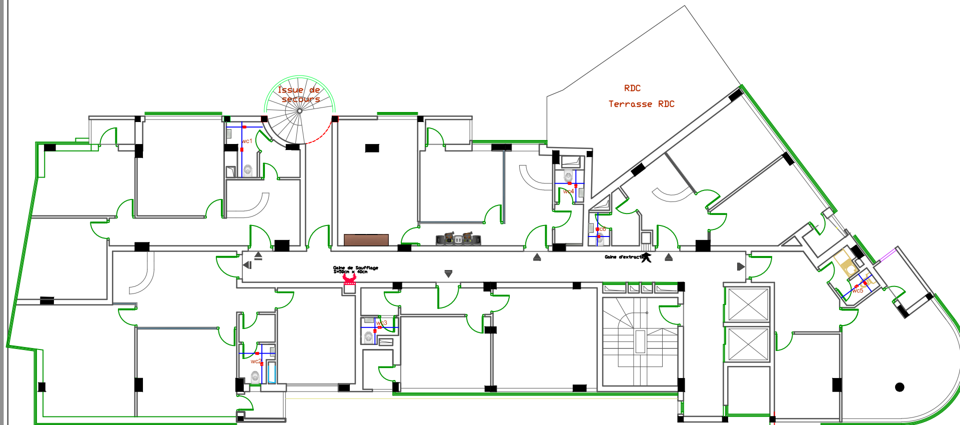
Plan courant: 1,2 ème Etage Ech: 1/100
